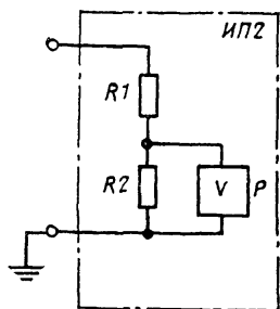
R_1 , R_2 —резисторы делителя; P —вольтметр
