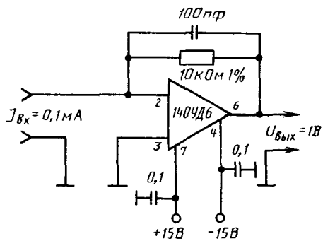
Схема технологического усилителя постоянного тока
