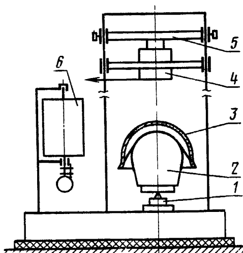
1—сидоизмерительный датчик; 2—макет головы; 3—каска; 4—ударник; 5—каретка; 6—фиксатор прогиба
