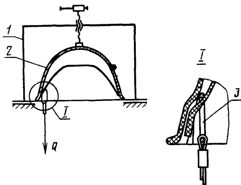
1—кронштейн; 2—каска; 3—захват
