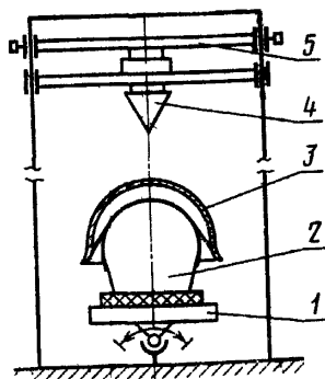
1—платформа; 2—макет головы; 3—каска; 4—конус; 5—каретка
