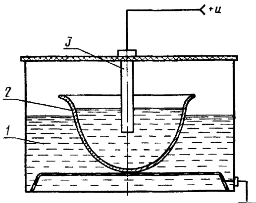
1—электролит, 2—корпус каски, 3—подвижной электрод
