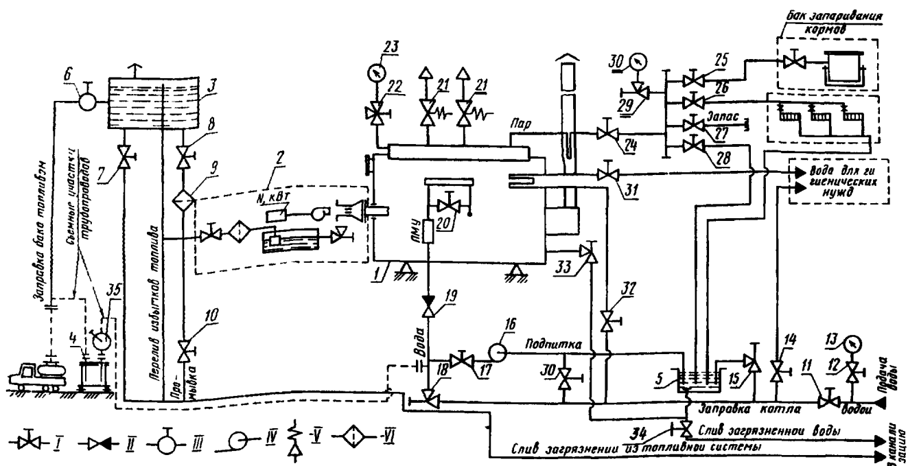
Схема котла КВ-300 М в сборе
