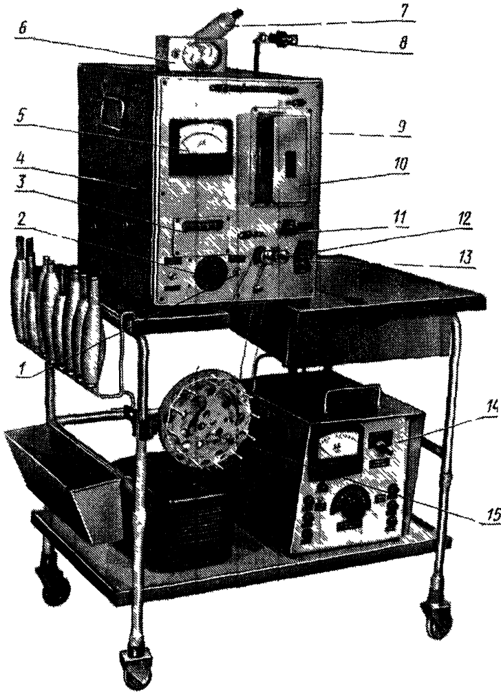
1—тумблер «двигатель включен», 2—ручка «регулировка усиления»; 3—счетчик метража, 4—ручка «установка счетчика на 0», 5—микроамперметр; 6—блок счета пороков, 7—шпудельдержатель; 8—нитенаправитель; 9—блок измерения; 10—датчик, 11—ручка «отвод ролика»; 12—приемный ролик; 13—переключатель «род работы», 14—блок питания 15—мотовило.
