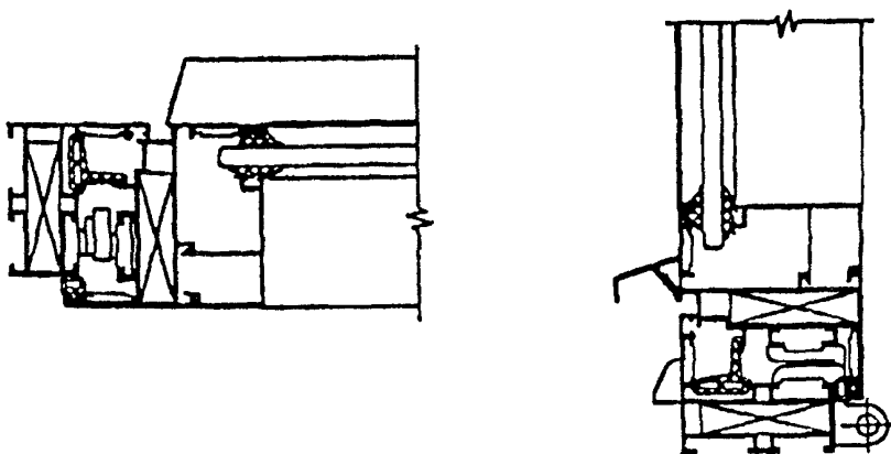
Рисунок 4 — Вариант конструктивного решения узлов притвора оконного блока с откидным открыванием внутрь помещения
