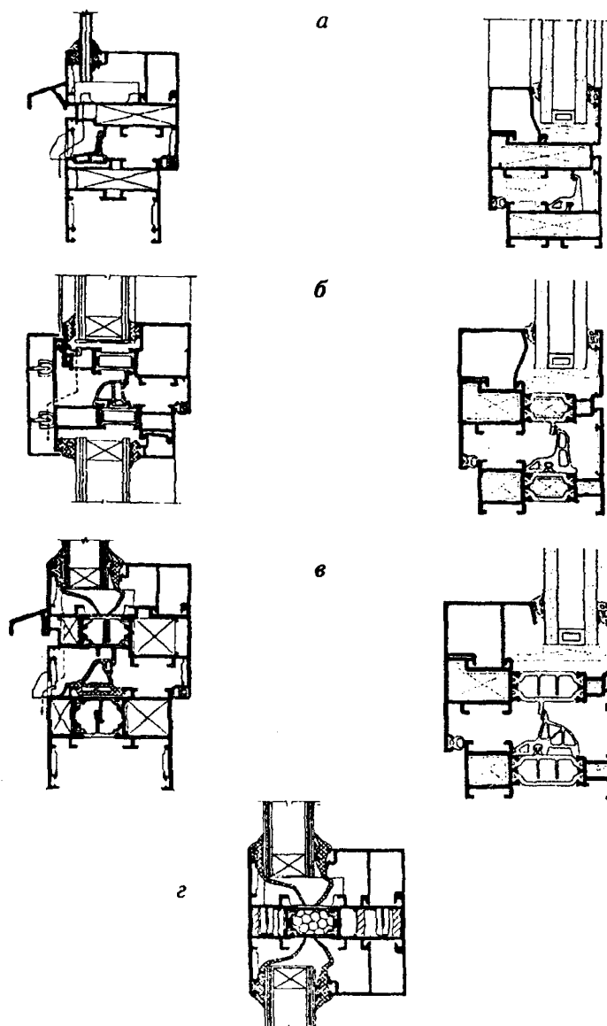
а — полые профили; б — комбинированные профили с однокамерной термоизоляционной вставкой; в — комбинированные профили с двух- и трехкамерной термоизоляционной вставкой; г — комбинированные профили с термоизоляционной вставкой, заполненной пенным утеплителем
