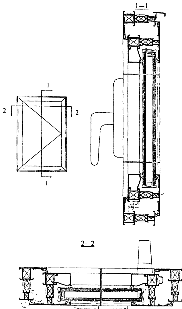
Рисунок 10 — Пример конструктивного решения балконного дверного блока с распашным открыванием наружу
