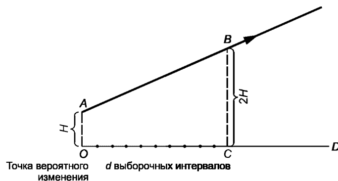
Рисунок Г.1 — Построение локальной разрешающей линии
