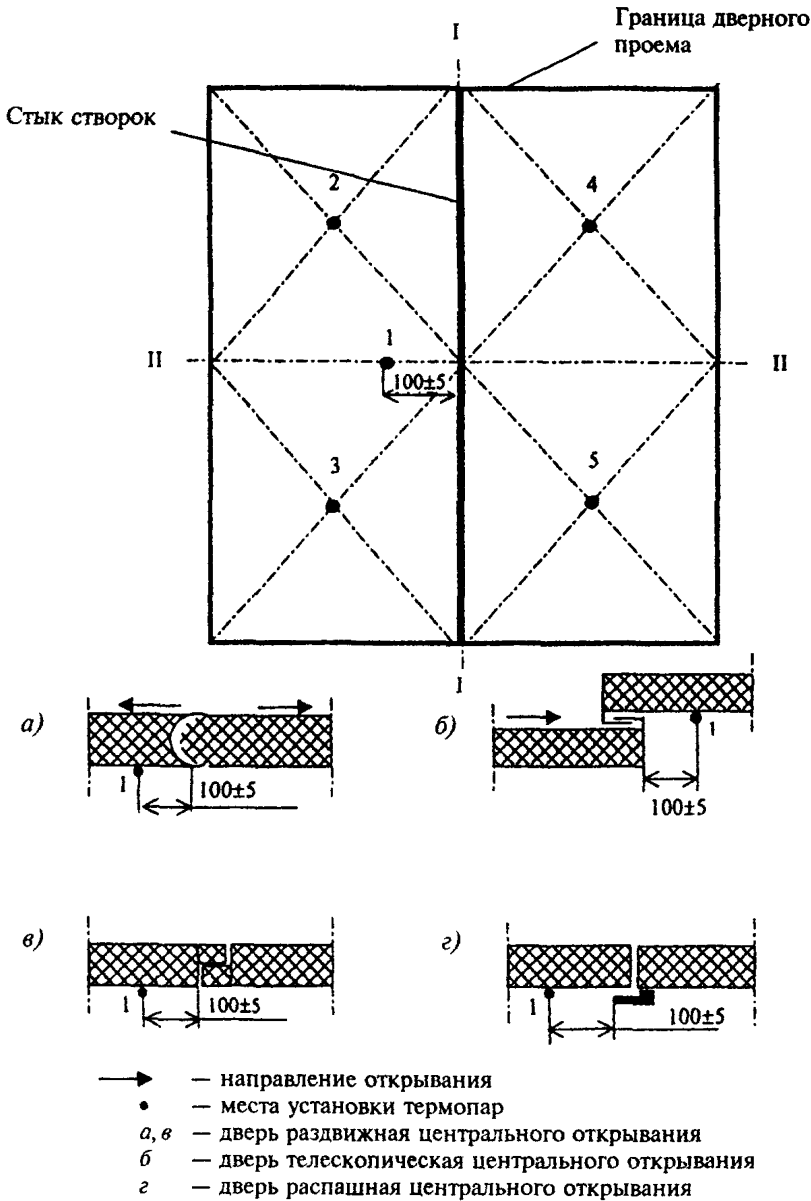
Рисунок А.2 — Схема установки термодпар на необогреваемой поверхности двухстворчатой двери
