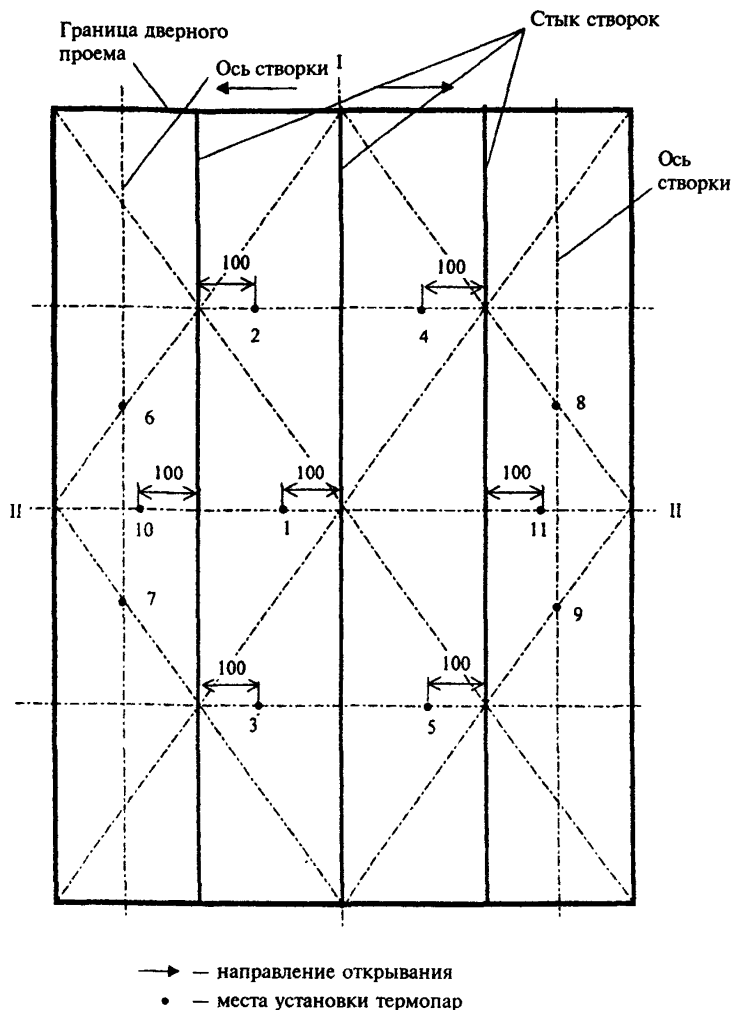
Рисунок А.4 — Схема установки термпар на неотапливаемой поверхности четырехстворчатой горизонтально-раздвижной двери центрального открывания
