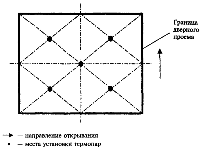
Рисунок А.7 — Схема установки термопар на необогреваемой поверхности вертикально-раздвижной одностворчатой двери
