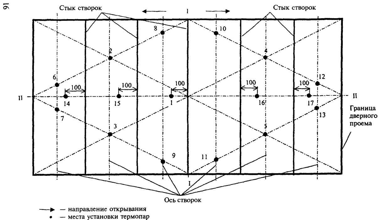
Рисунок А.5 — Схема установки термопар на необогреваемой поверхности шестистворчатой горизонтально-раздвижной двери центрального открывания
