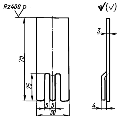
Подвеска П2
