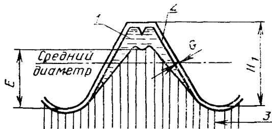
1—частичное обезуглероживание; 2—полное обезуглероживание; 3—основной металл; H_1 —высота профиля наружной резьбы. Значения H_1 приведены в табл. 12.
