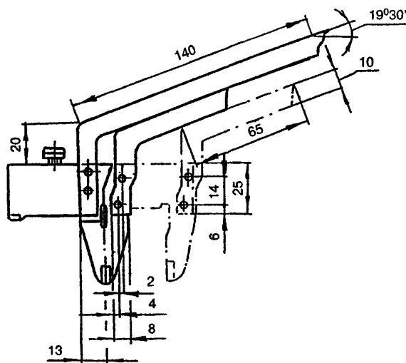
Рисунок 3 — Передвижной шаблон
