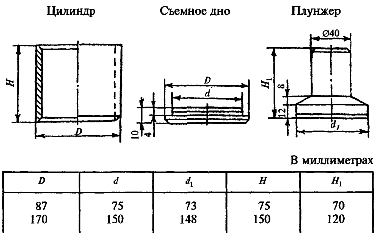
Рисунок 4 — Цилиндры стальные
