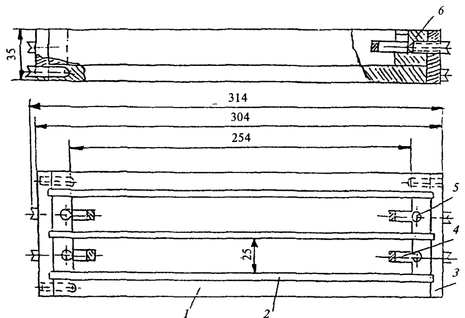
Рисунок 12 — Форма для изготовления образцов-балочек
