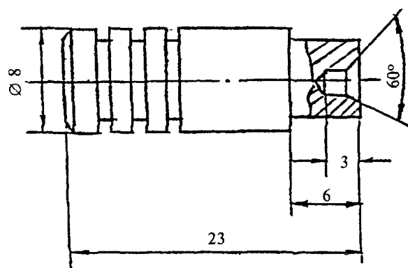
Рисунок 13 — Репер для испытаний
