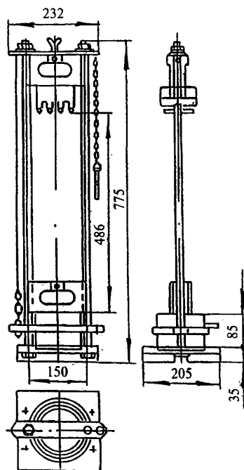
Рисунок 7 — Копер ПМ
