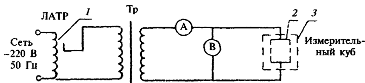
1 — лабораторный регулировочный трансформатор (ЛАТР); 2 — электрод; 3 — измерительный куб
