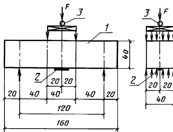
Схема нагружения опытного образца
