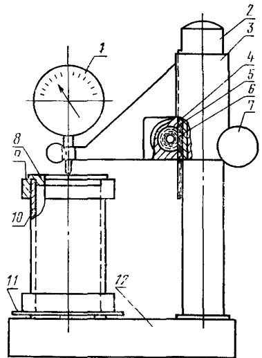
Прибор ГОИ
