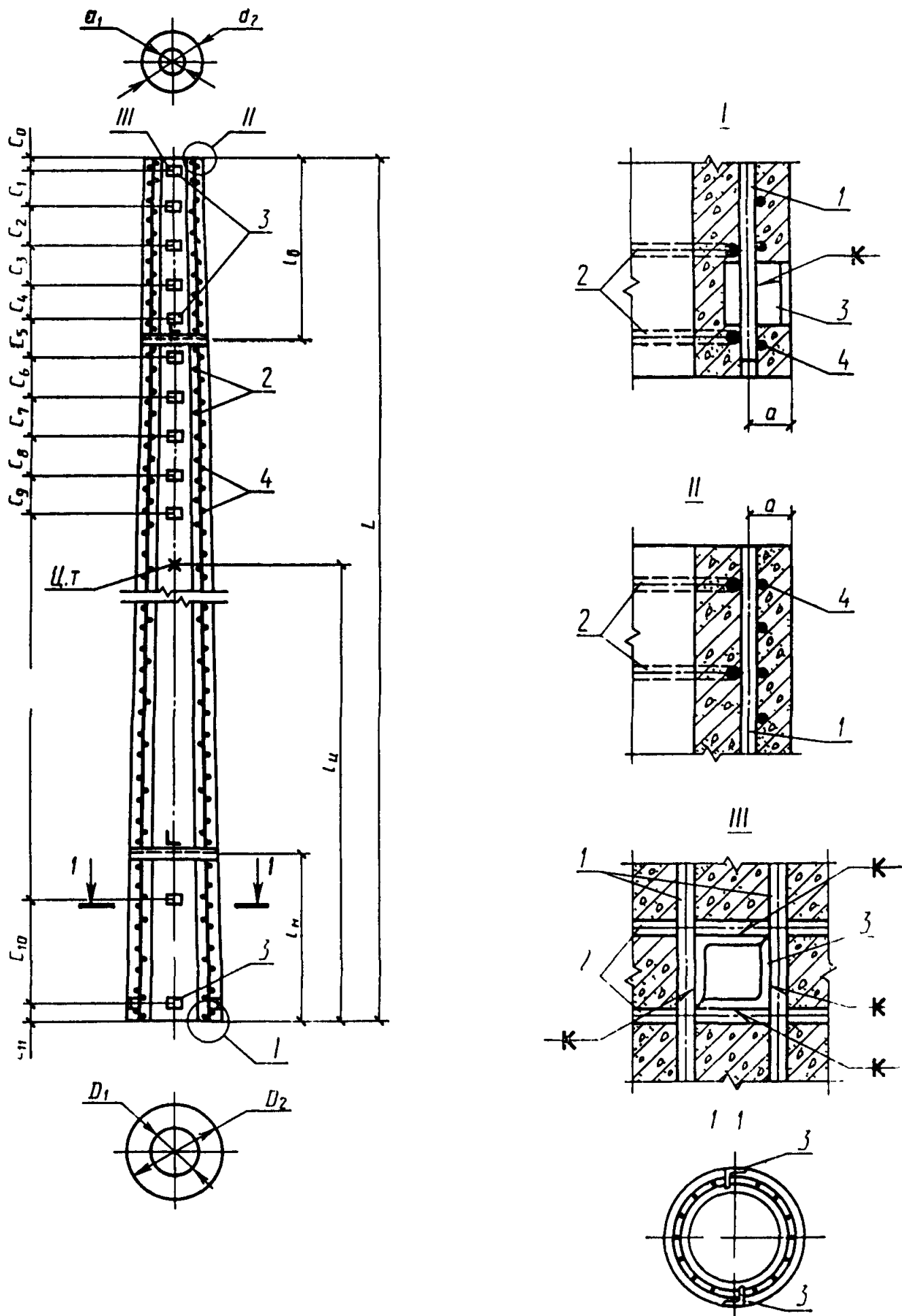
1—продольная арматура, 2—монтажные кольца, 3—закладные изделия, 4—спираль; a —расстояние от наружной поверхности стойки до оси продольной арматуры, c_0 — c_{11} —вязка закладных изделий, ц.т.—центр тяжести; L —длина стойки, l_{ц} —расстояние до центра тяжести, l_{н} , l_{в} —расстояния от мест установки диафрагм, D_1 , d_1 —внутренние диаметры стойки, D_2 , d_2 —наружные диаметры стойки
