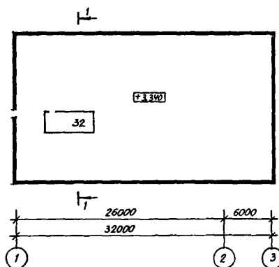
ПЛАН ЧЕРДАКА
