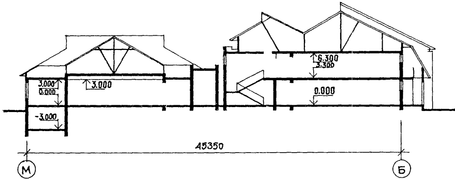
РАЗРЕЗ I-I
