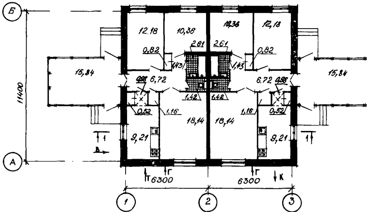
ПЛАН
