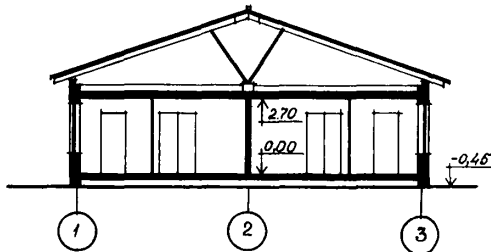
РАЗРЕЗ I-I
