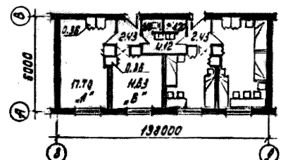
ФРАГМЕНТ ПЛАНА В ОСЯХ 8-9
