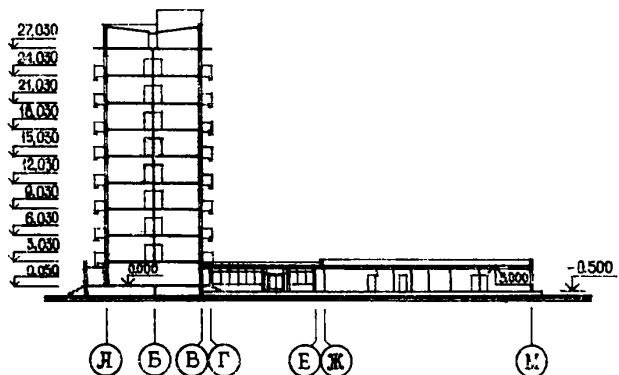
РАЗРЕЗ Б-Б
