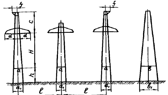
ДУХУЦЕПНАЯ КОНЦЕВАЯ ОПОРА
